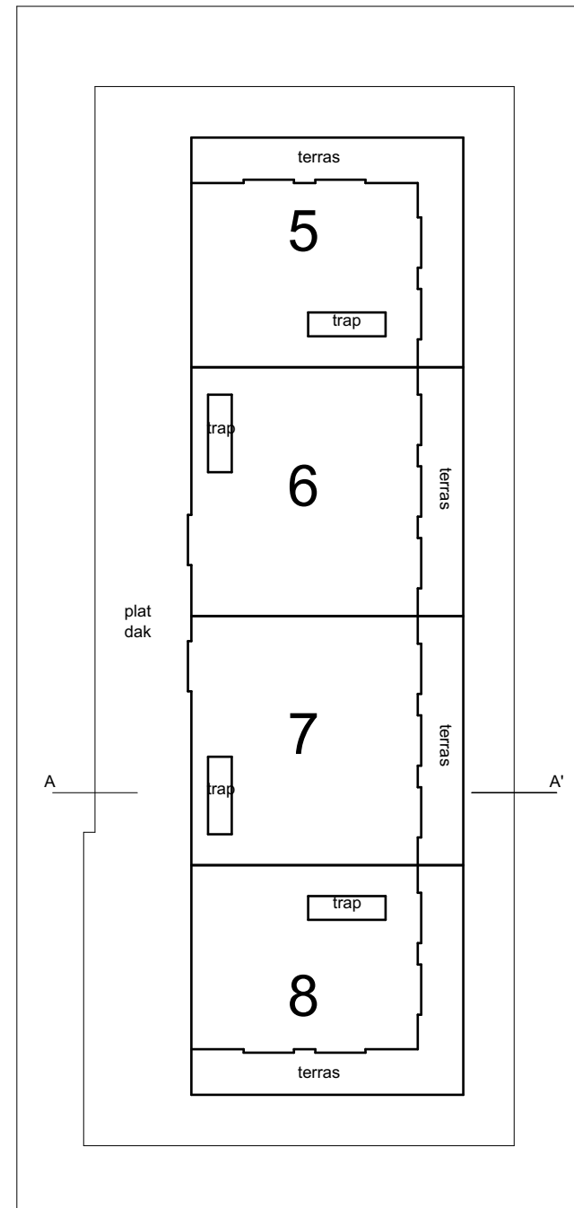
3e verdieping 1:200
