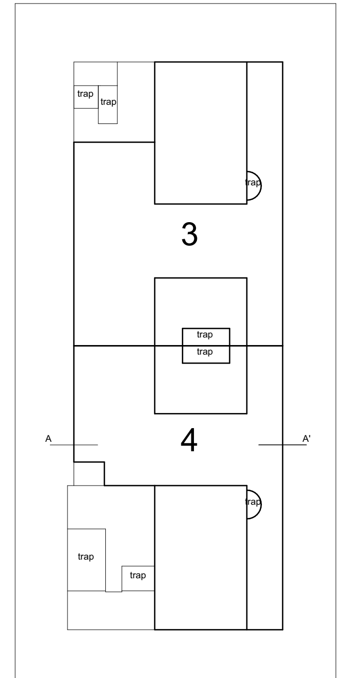
entresol 2 1:200
