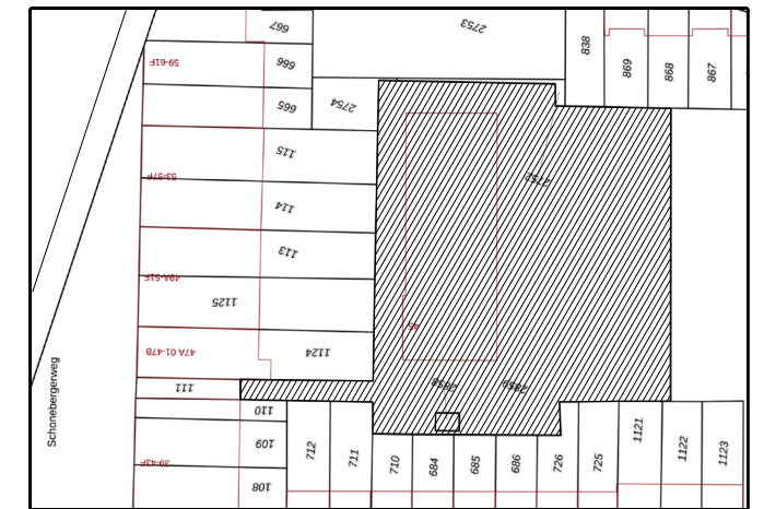
situatie 1:1000
